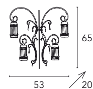
Casanova 1881/A4L 4 x max 60W E14 230V CE V
