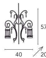
Casanova 1881/A2L 2 x max 60W E14 230V CE V
