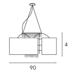
Onda 2113/L4L 4 x max 60W E14 230V CE V
