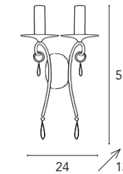
Sinfonia 3019/A2L 2 x max 60W E14 230V CE V A B
