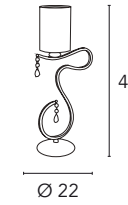
Delhia 2015/LU 1 x max 60W E14 230V CE V
