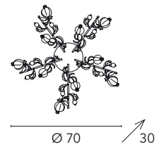
Ametista 1650/PL10L 10 x max 40W G9 230V CE V R ⊕
