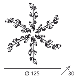
Ametista 1650/PL18L 18 x max 40W G9 230V CE V R ⊕
