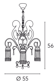
Casanova 1881/L3L 3 x max 60W E14 230V CE V
